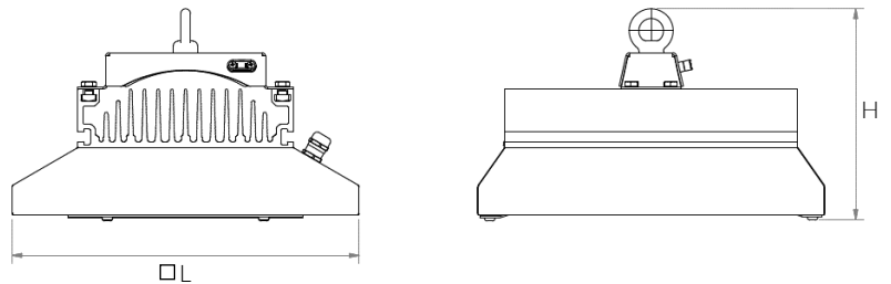
SPACE-S + UCHWYT-G-SPACE-I
